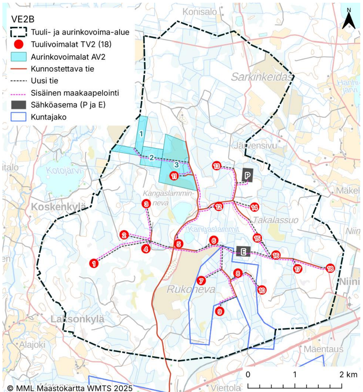
Kuva 2. Kangaslammin tuulivoimapauston alustava voimalasijoittelu vaihtoehdossa VE2B, 18 tuulivoimalaa ja 99 ha aurinkovoimaa. Kaavaluonnos pohjautuu YVA:n vaihtoehdolle VE2B.
